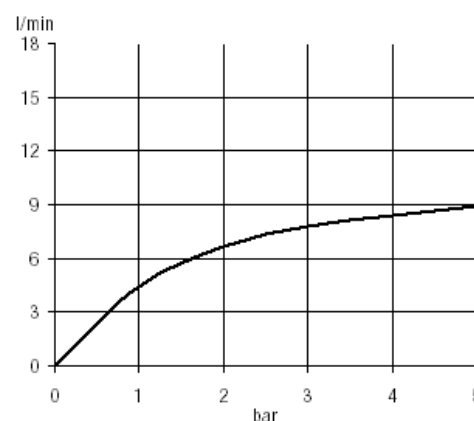
Diagram przepływu
