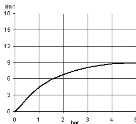
Diagram przepływu
