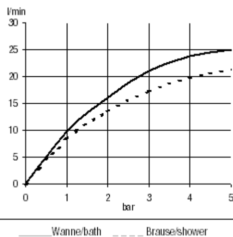
Diagram przepływu
